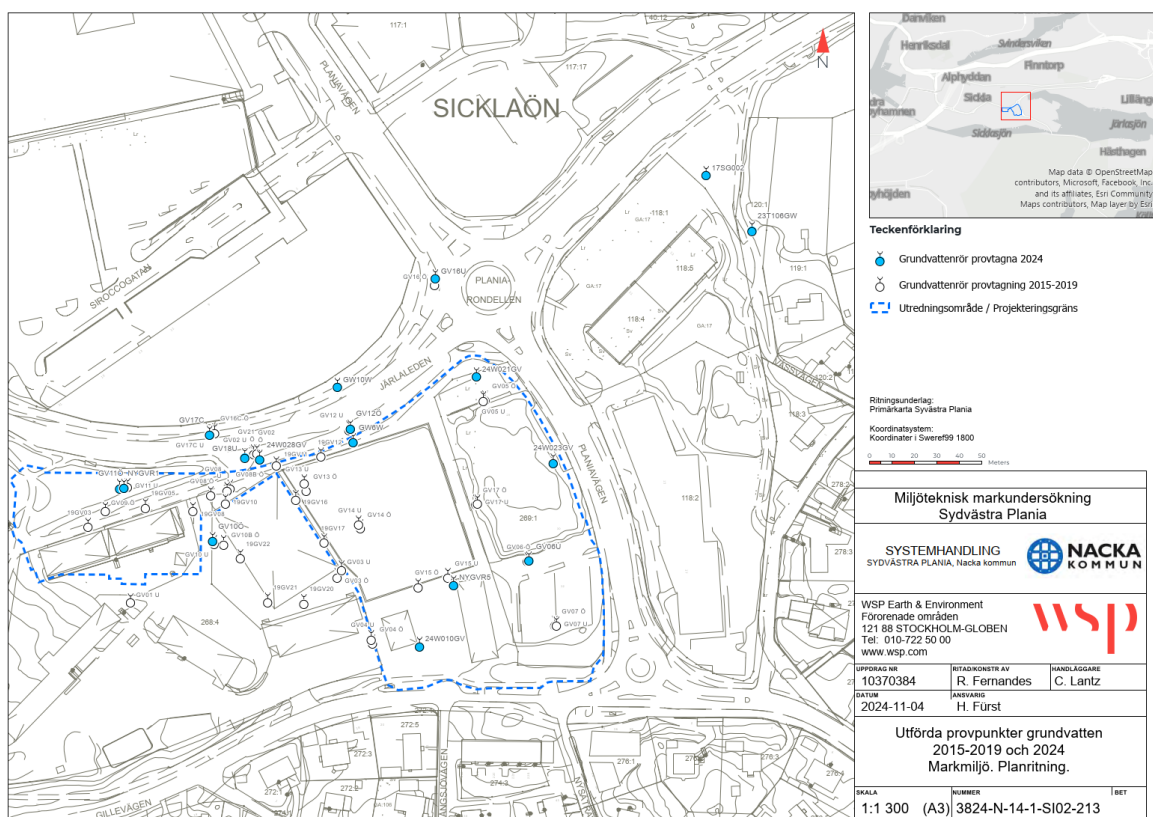
Figur 28 Ritning som visar provpunkter för grundvatten inom och utanför planområdet. Blå streckad linje utgör utredningsområde. Ofyllda tecken markerar grundvattenrör provtagna 2015-2019. Blå fyllda tecken visar grundvattenrör provtagna 2024. Källa: (WSP, 2024b).
